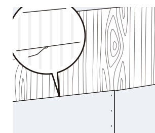
せっこうボードと合板の取り合い
